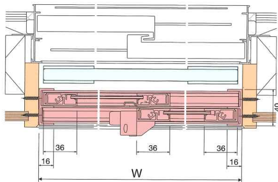
[ 横断面納まり図 ]
