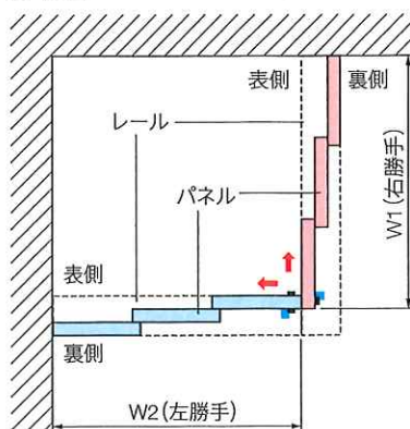
見下げ図
